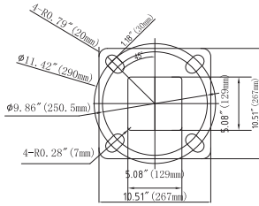
5" Flange
